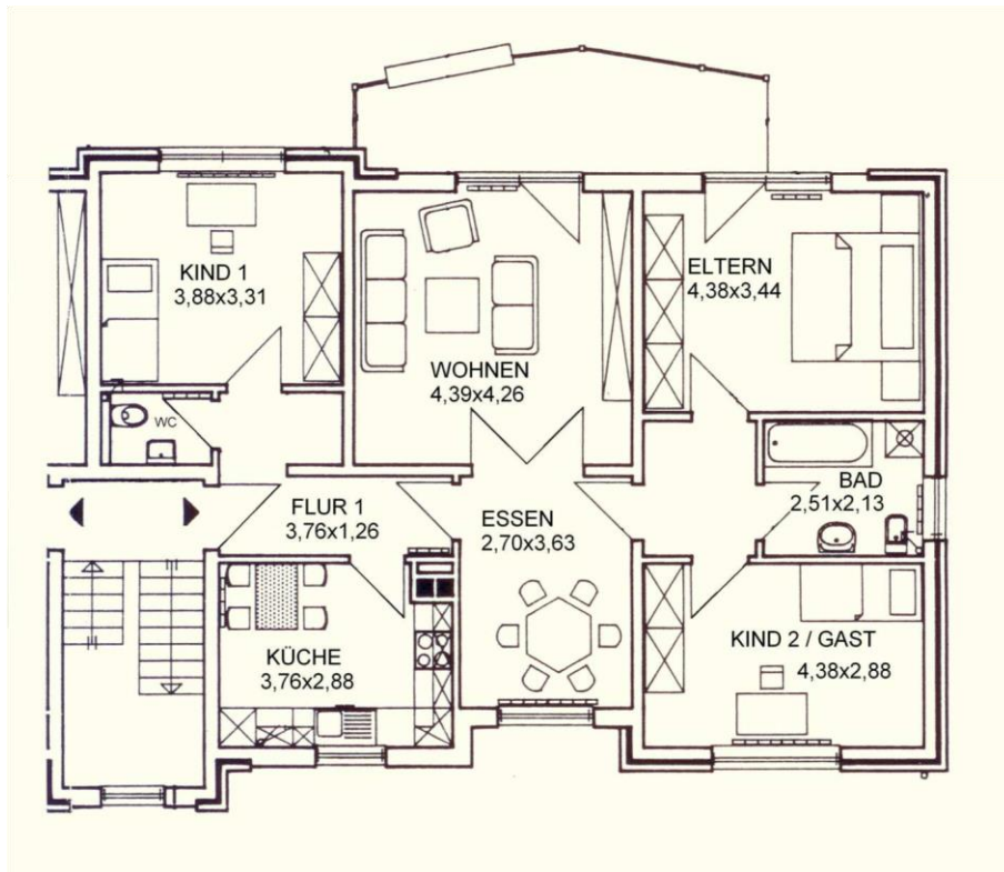
Mehrfamilienhaus (Typ D) 4-Raum-Wohnung
