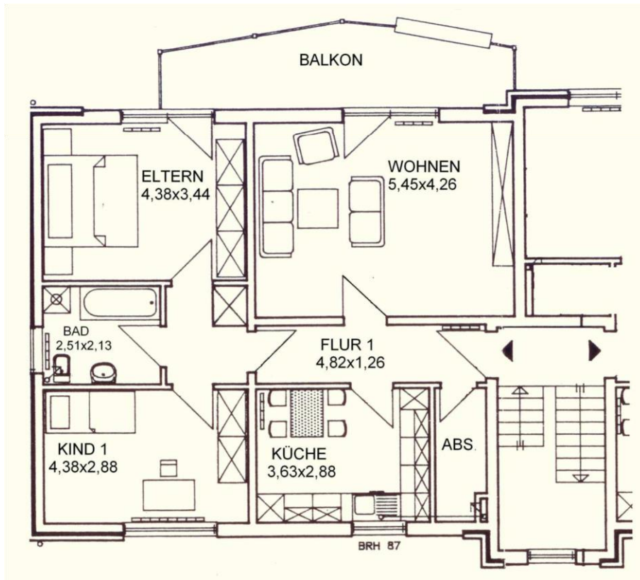
Mehrfamilienhaus (Typ D) 3-Raum-Wohnung
