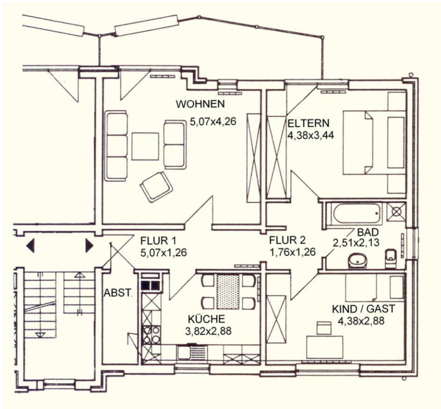
Mehrfamilienhaus (Typ E) 3-Raum-Wohnung
